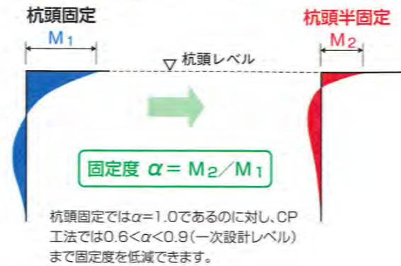
杭曲げモーメント分布
