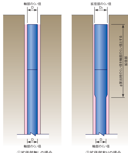
ψ算定時におけるくい径
