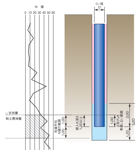
くい先端適用範囲
