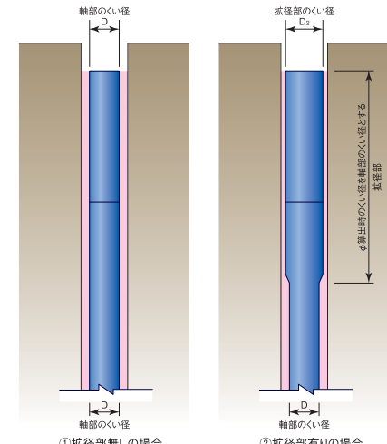
ψ算定時におけるくい径
