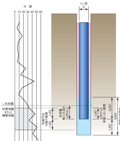
くい先端適用範囲
