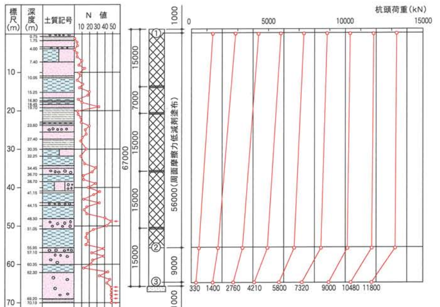
軸力分布図
